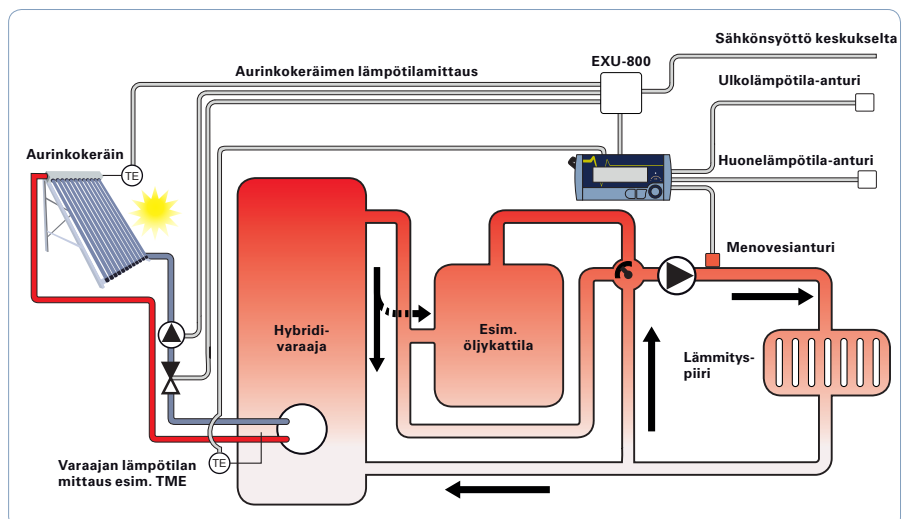
Periaatekuva hybridilämmityksestä, jossa lämmönsäädin ohjaa aurinkokeräimen ja varaajan välistä latauspumppua ja -venttiiliä sekä toimii lämmitysjärjestelmän säätimenä ulkolämpötilan ja menoveden lämpötilan perusteella.
