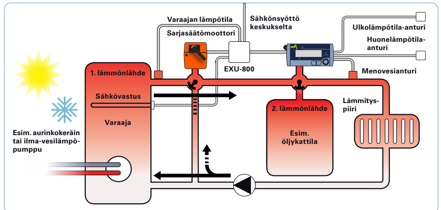
Periaatekuva hybridilämmityksestä, jossa sarjasäätömoottori ottaa tehoa 1. lämmönlähteestä. Kun 1. lämmönlähteestä loppuu teho, säädin alkaa ottaa lisätehoa 2. lämmönlähteestä. Pintalämpötila-anturi on kytketty mittaamaan (1. lämmönlähteen) varaajan lämpötilaa.
